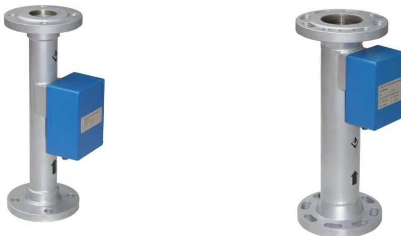
Рисунок 1 - Первичный измерительный преобразователь влагомеров ВСН-2-50 и ВСН-2-80 в прямоточном исполнении
