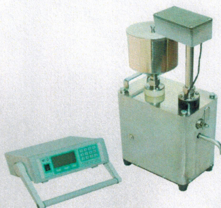
Рисунок 1 – Общий вид влагомеров сырой нефти лабораторных ВСН-Л-01 и ВСН-Л-02
