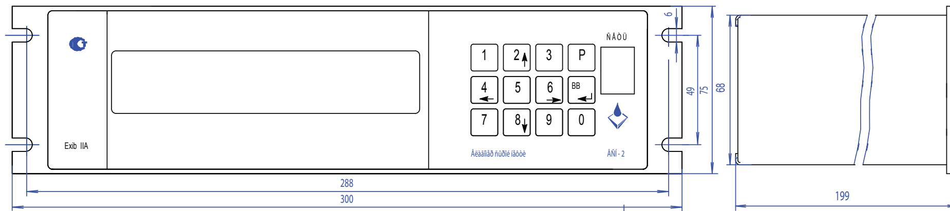
Чертеж узла крепления прибора в стойке
