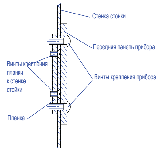
Чертеж узла крепления прибора в стойке
