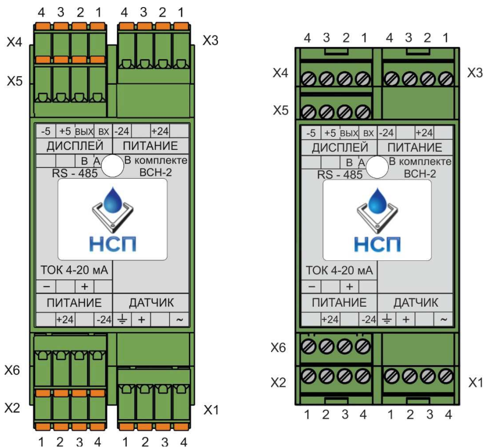
Рис 5. Вариант исполнения с графическим дисплеем.
