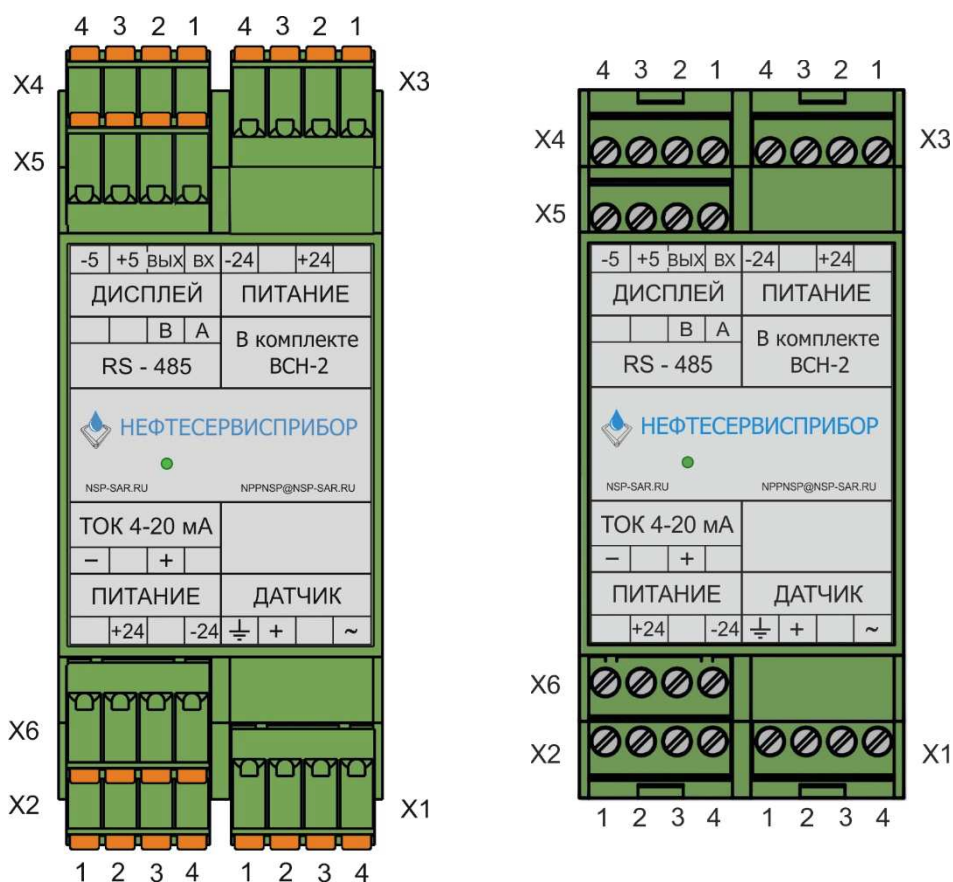
Рис 4. Основной вариант исполнения
